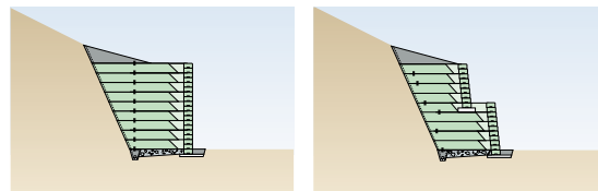
TerraBloc® mit Erdbewehrung, Frontneigung 90° oder Anzug 8:1
